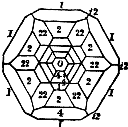
Vesuvius.
